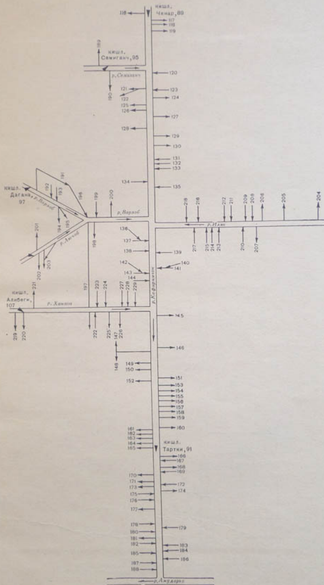
Рис. 5. Схема расположения водозаборов, коллекторов и сбросов в бассейне р. Кафиринжан.
