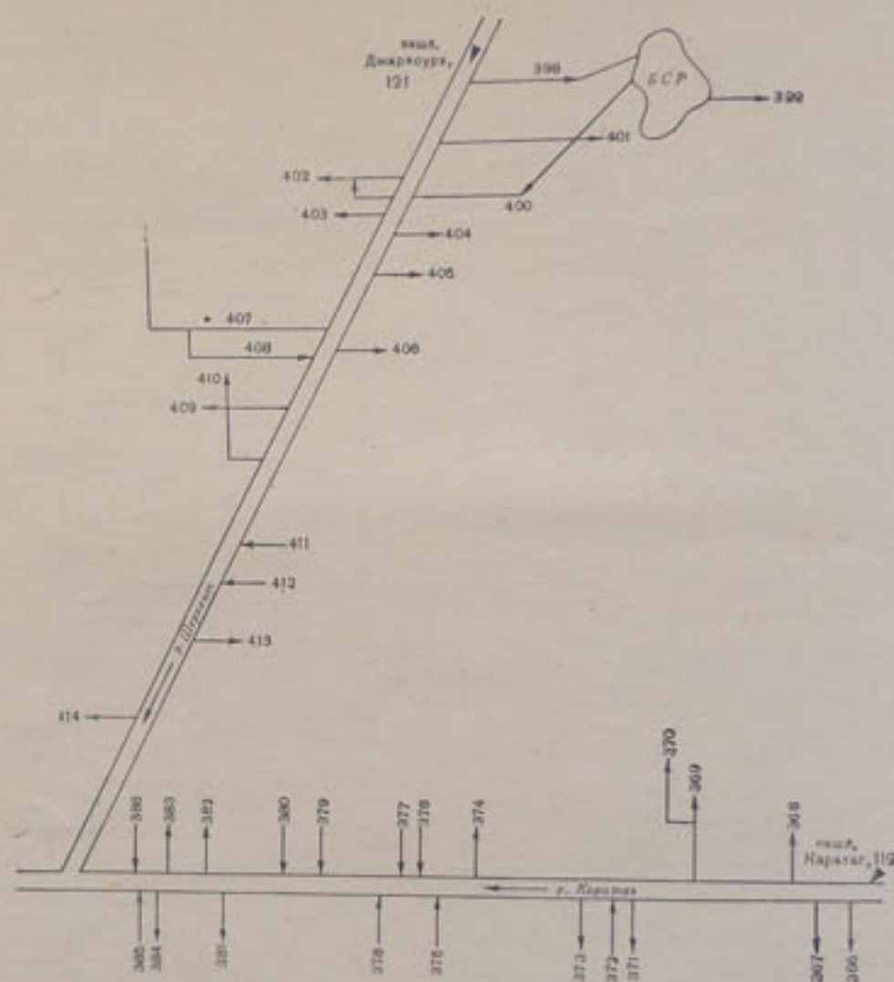
Рис. 8. Схема расположения водозаборов, коллекторов и сбросов в бассейнах рек Каратаг и Шеркент.
