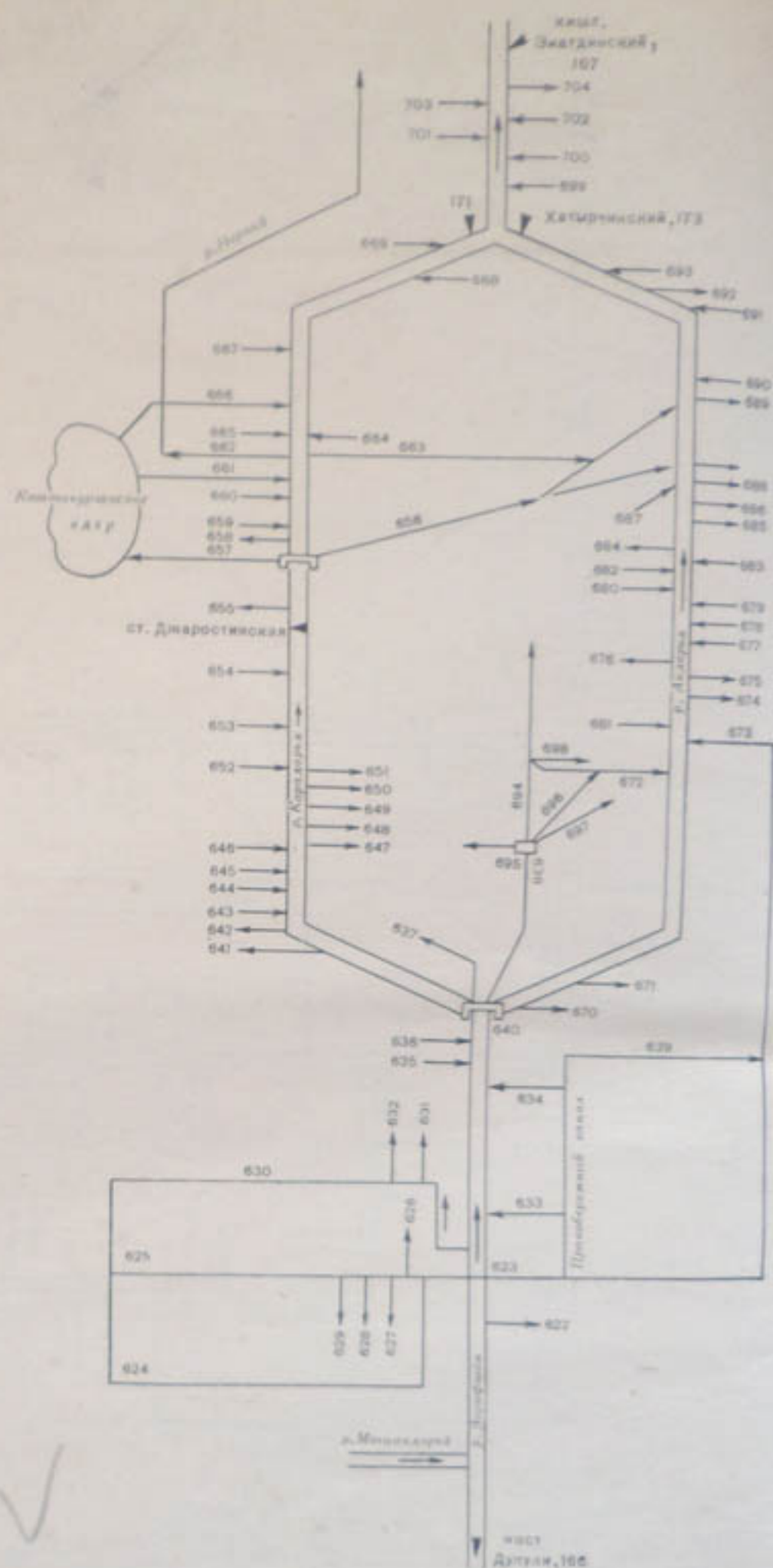
Рис. 11. Схема расположения водозаборов и сбросов в бассейне р. Зарафшан (нижнее течение).
