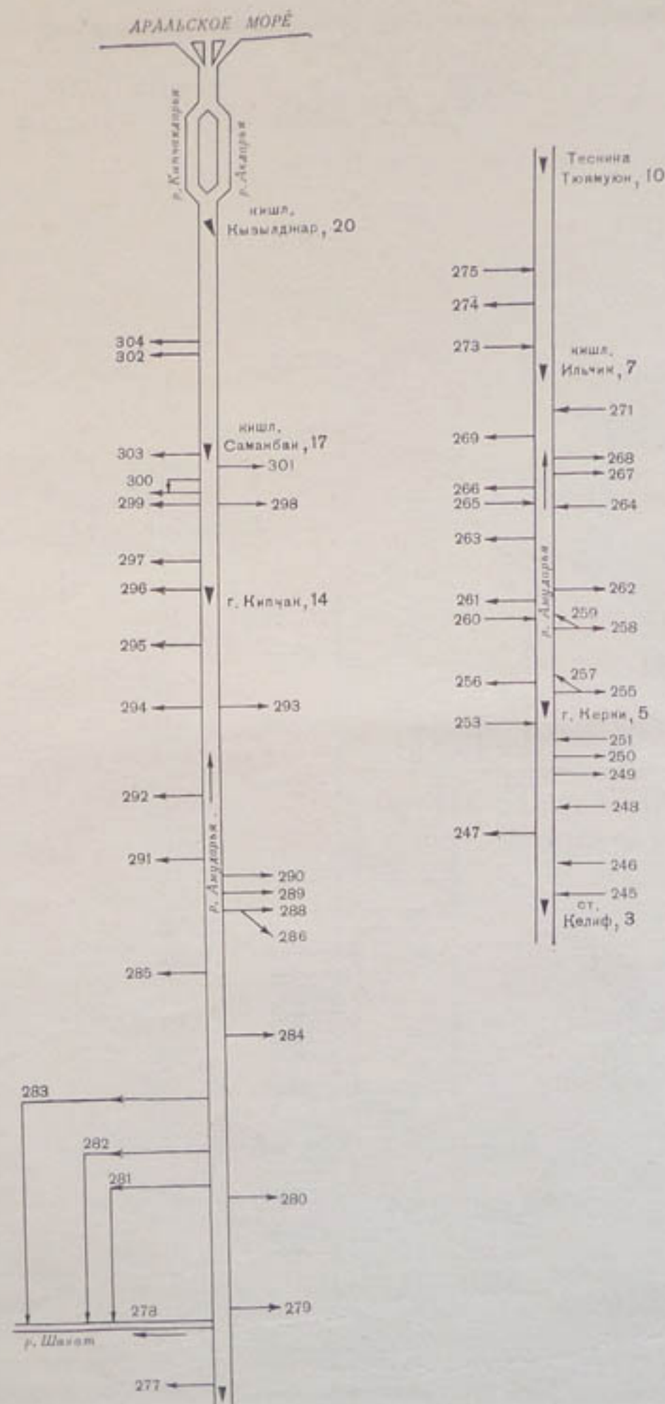
Рис. 6. Схема расположения водозаборов, сбросов и коллекторов в бассейне р. Амударья от ст. Келиф до Аральского моря.
