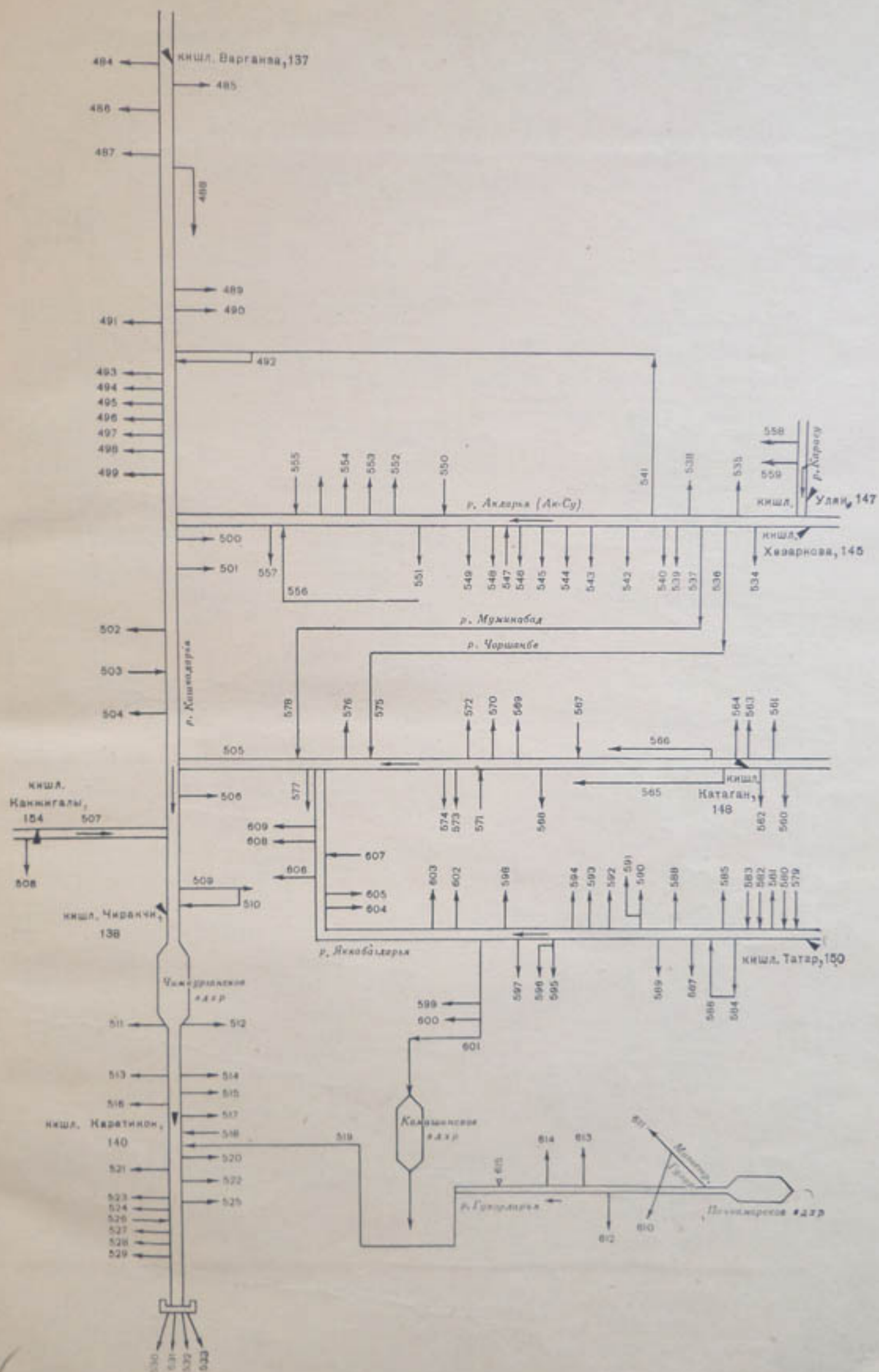
Рис. 9. Схема расположения водозаборов и сбросов в бассейнах рек Кашкадарья, Жандыдаарья, Акдарья, Танхиздаарья, Якабадаарья и Гузардаарья.
