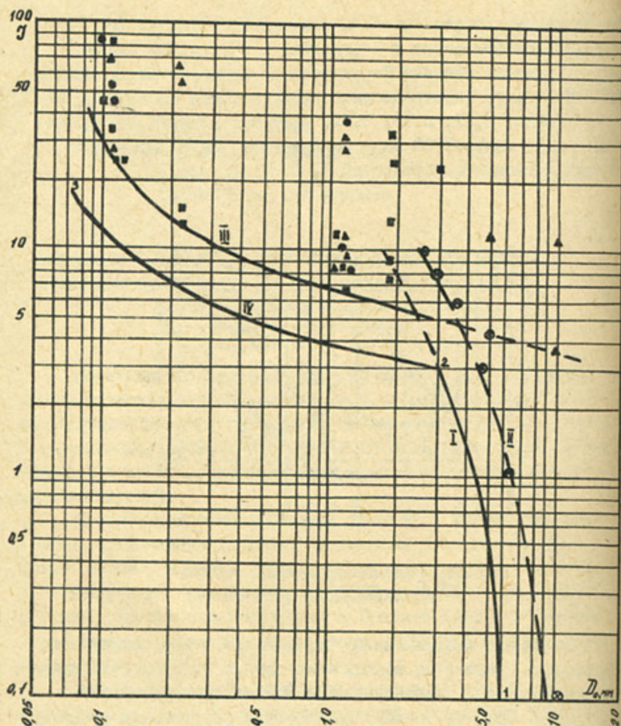
Рис.2. Зависимости градиентов напора от диаметра фильтрационного хода: I – теоретическая и II – опытная расчетные кривые ( \odot – опытные точки) Г.Х.Праведного для пластичных грунтов, III – опытная и IV – расчетная кривые для слабосвязных грунтов ( \odot , \blacktriangle , \blacksquare – опытные точки, соответствующие начальным плотностям супесей – 1,5; 1,6; 1,7 т/м 3 ).
