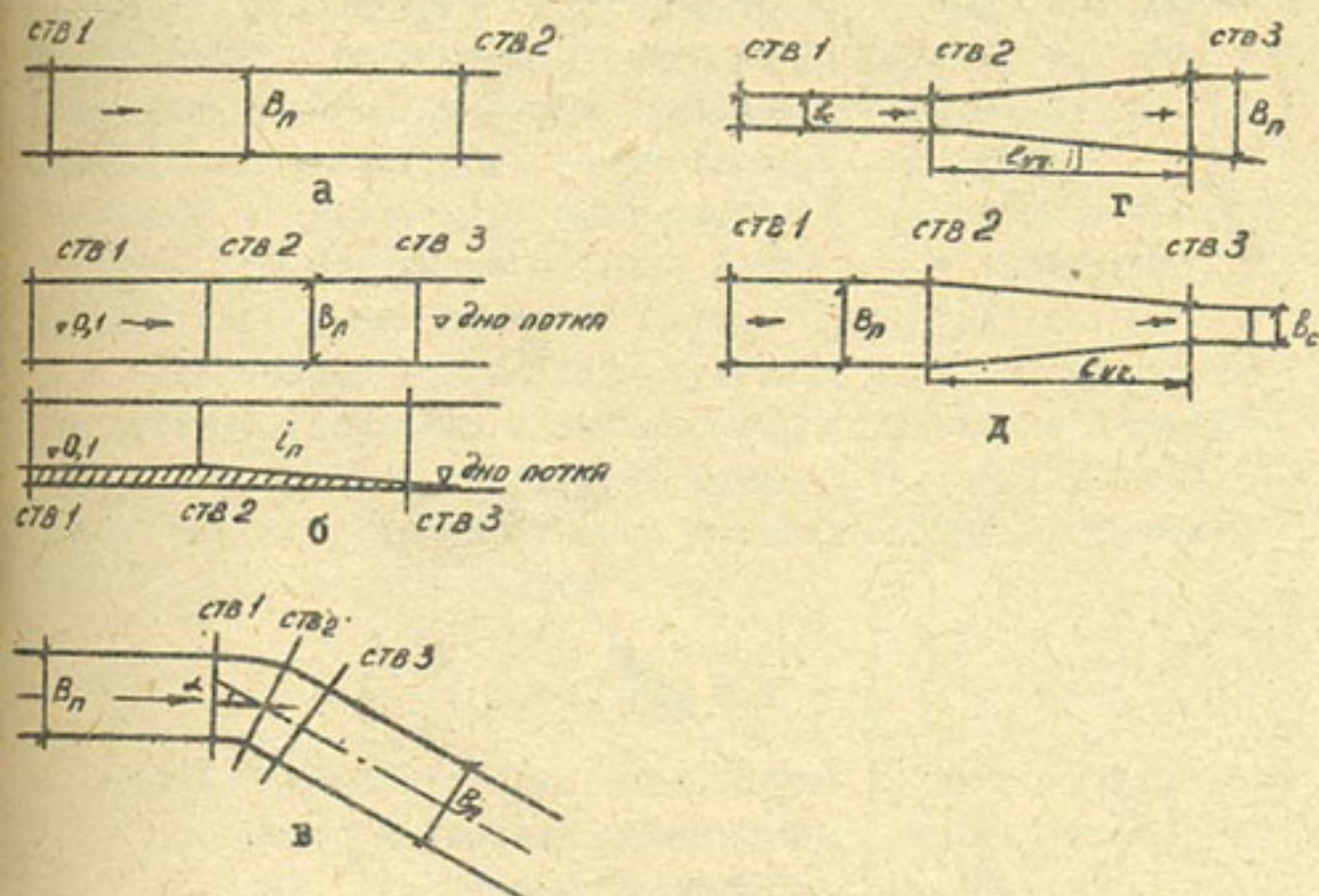
Рис. I. Схемы экспериментальных установок: а — постоянная ширина B_n = const ; б — при уклонах дна i_n = 0,05; 0,07; 0,1 ; в — при изменении направления течения под углом \alpha = 30^\circ; 50^\circ; 70^\circ ; г и д — при расширении и сужении потока в пределах
